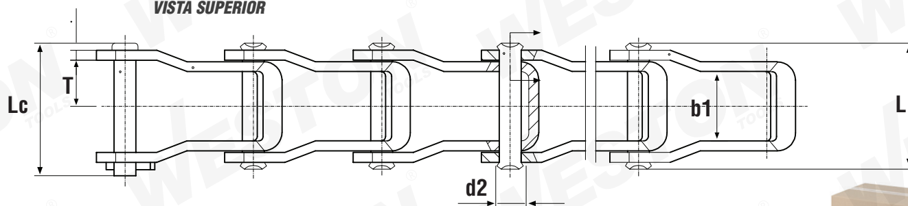
VISTA SUPERIOR
